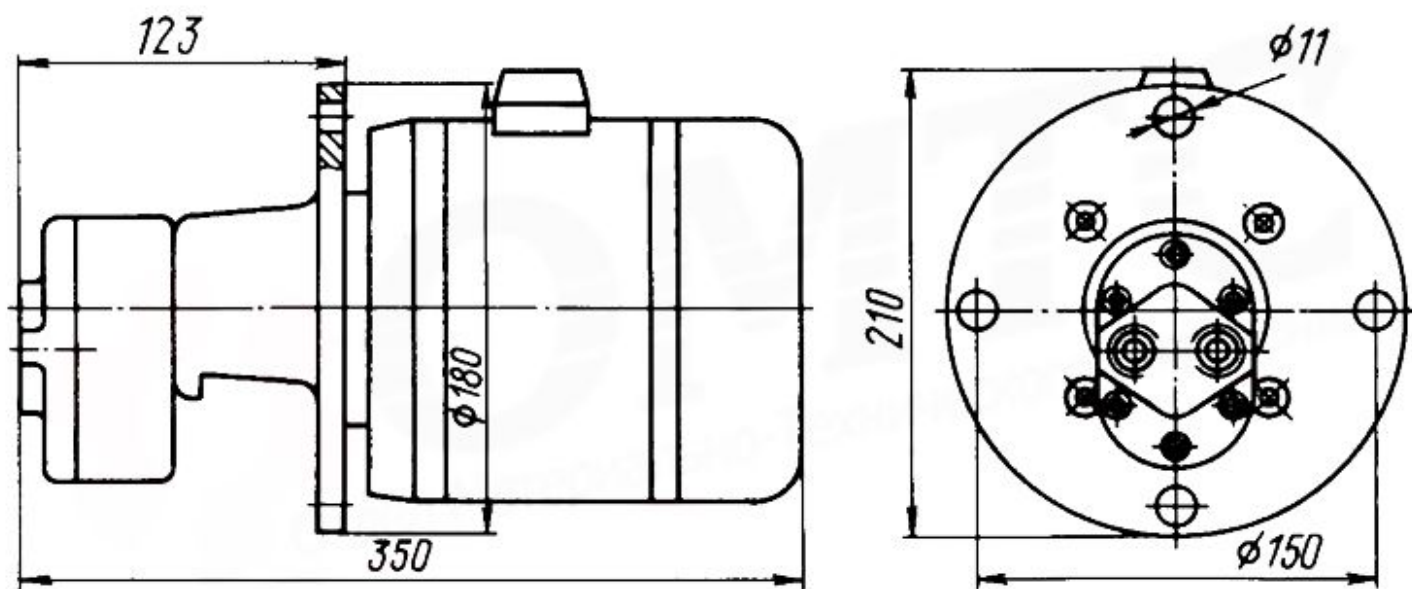
ВГ11-1 с двигателем ДПТ 21-4, АОЛ 21-4
