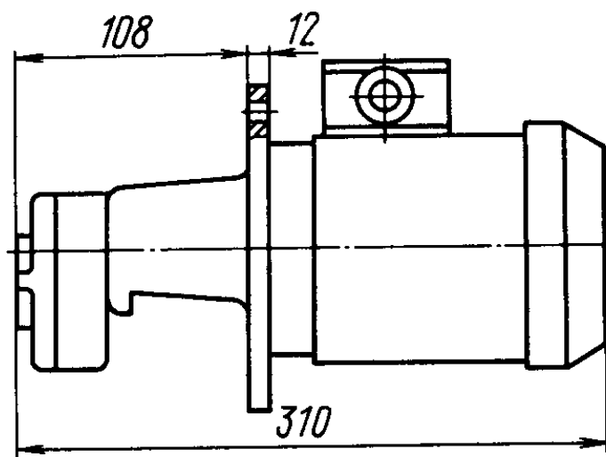
БГ11-1 с двигателем 4АА63
