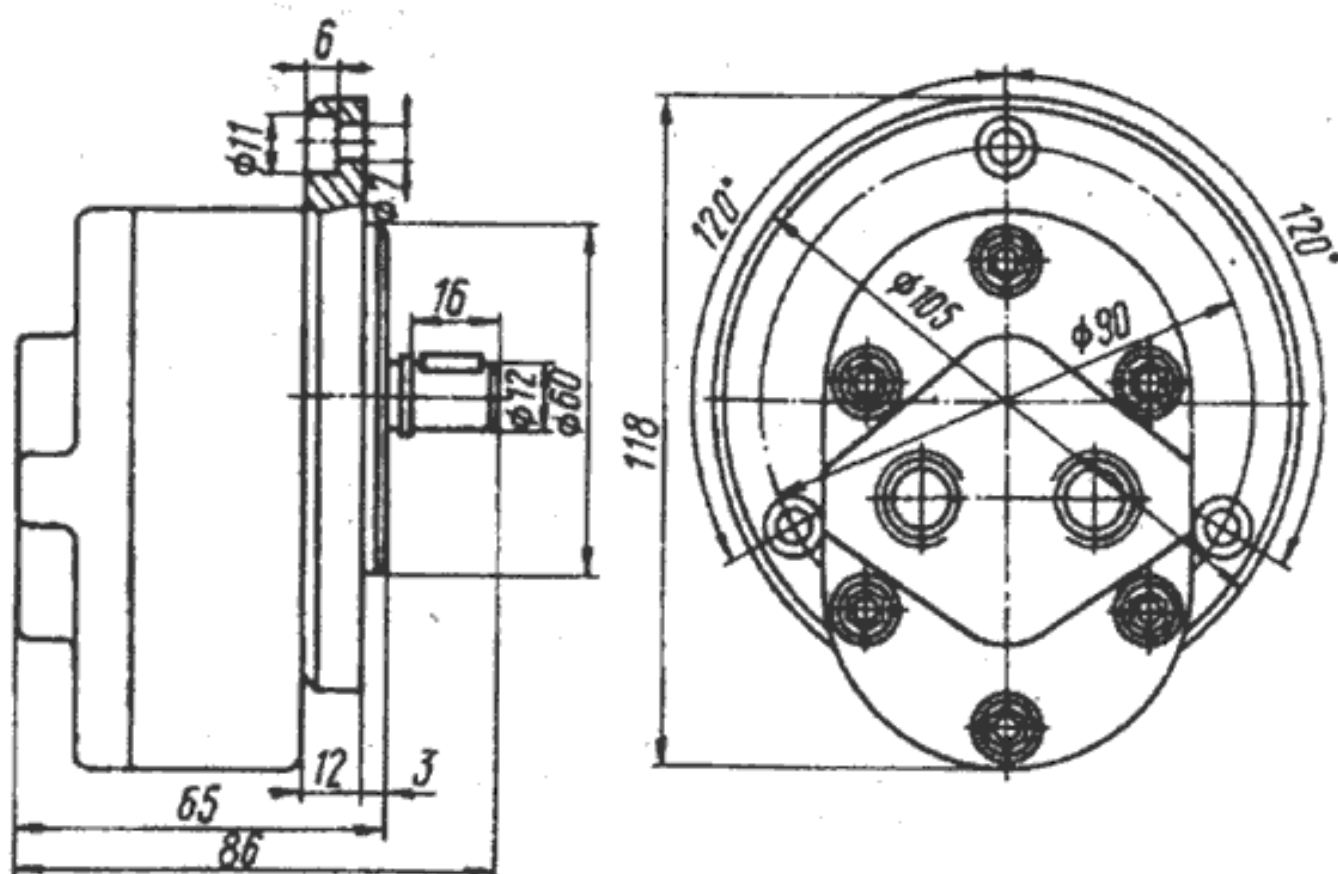
Габаритные и присоединительные размеры насосов АГ11-1
