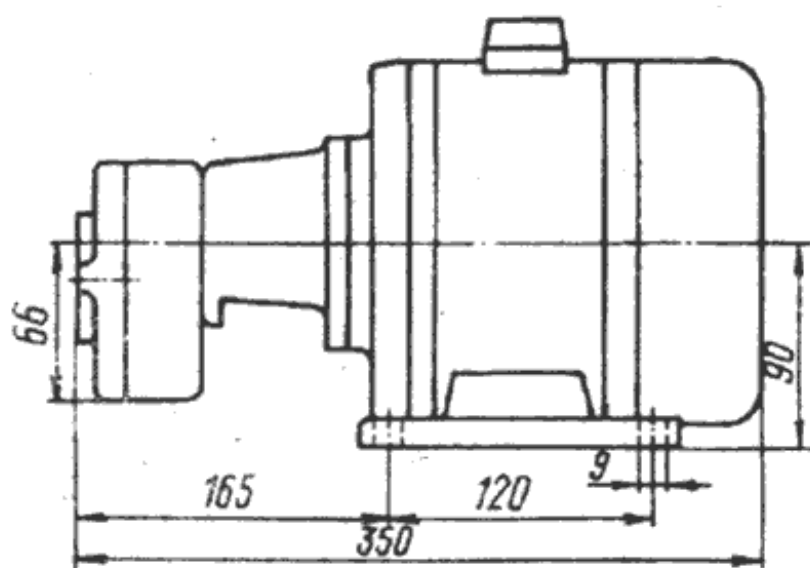
Габаритные и присоединительные размеры насосных агрегатов БГ11-1 с двигателем серии ДПТ 21-4 или АОЛ 21-4
