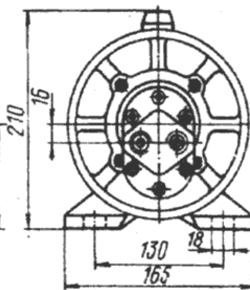
Габаритные и присоединительные размеры насосных агрегатов БГ11-1 с двигателем серии ДПТ 21-4 или АОЛ 21-4
