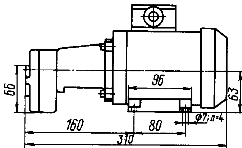
БГ11-1 с двигателем 4АА63
