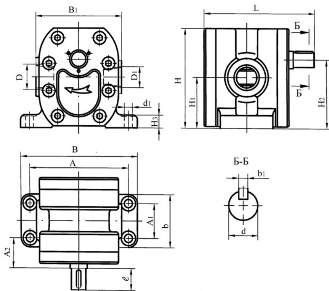
Габаритные и присоединительные размеры насосов Г11-2
