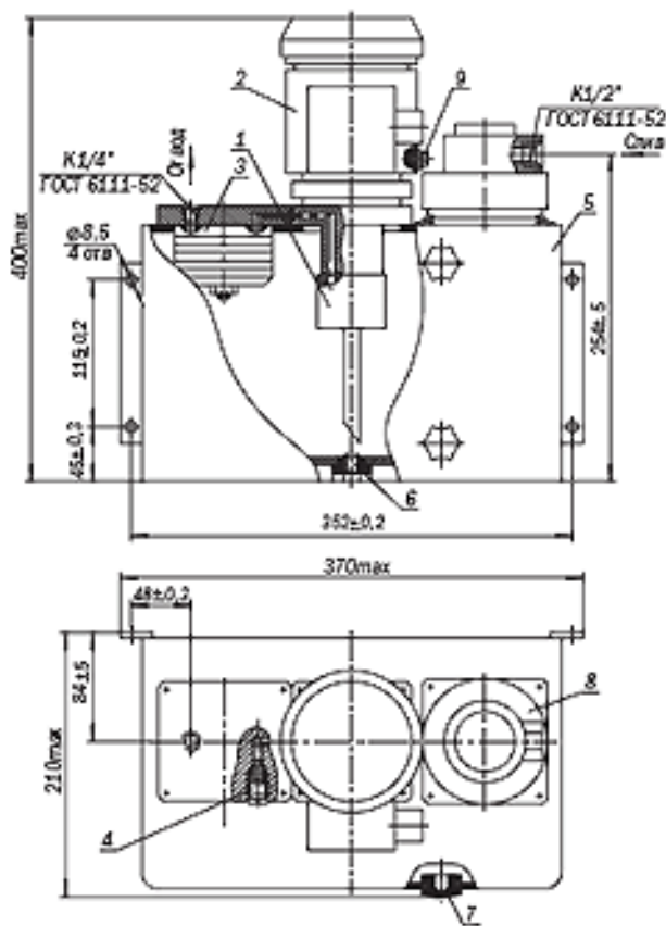
Рис.1. Станция смазочная типа С48-1М.
