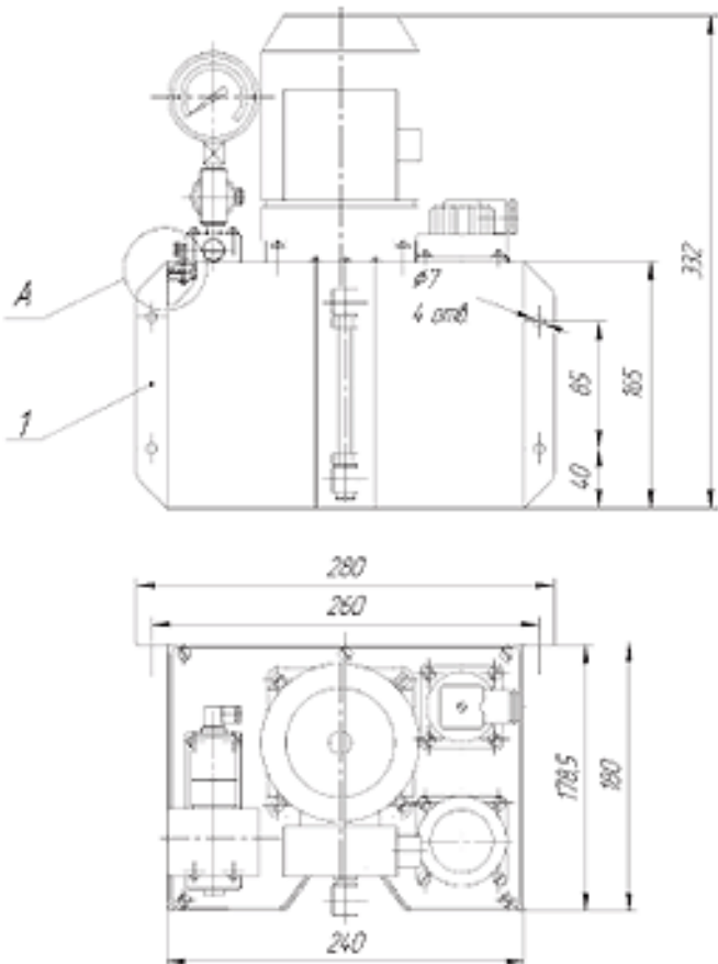
Рис.2. Станция смазочная типа МС48М.
